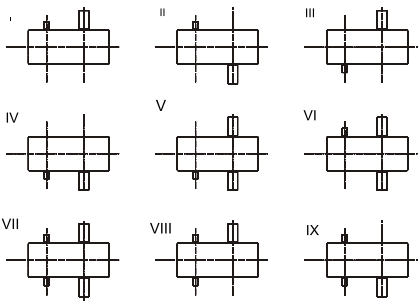
POSICIONES DE MONTAJE
